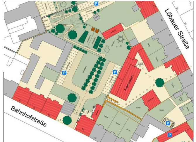
Lageplan zur Freiflächen- gestaltung
