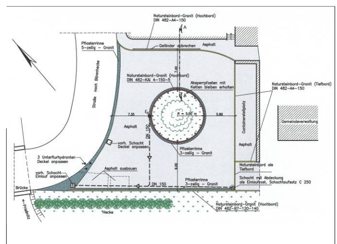
Gestaltungsplan
